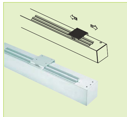
Flexible Montagewinkel
